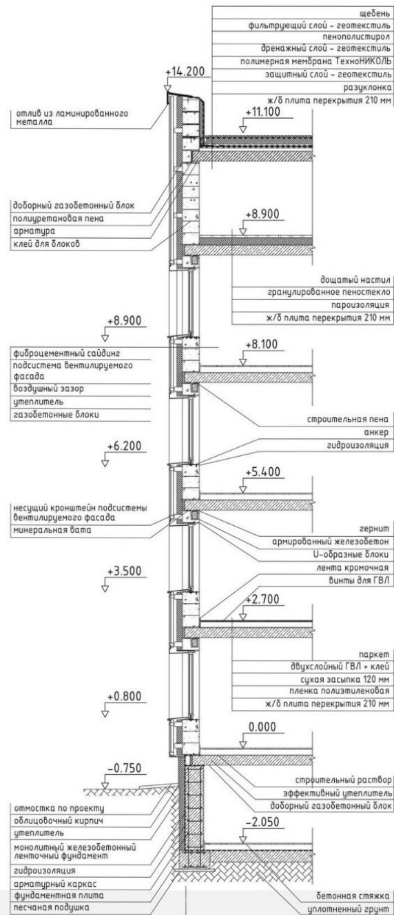
Разрез по стене М 1:50
